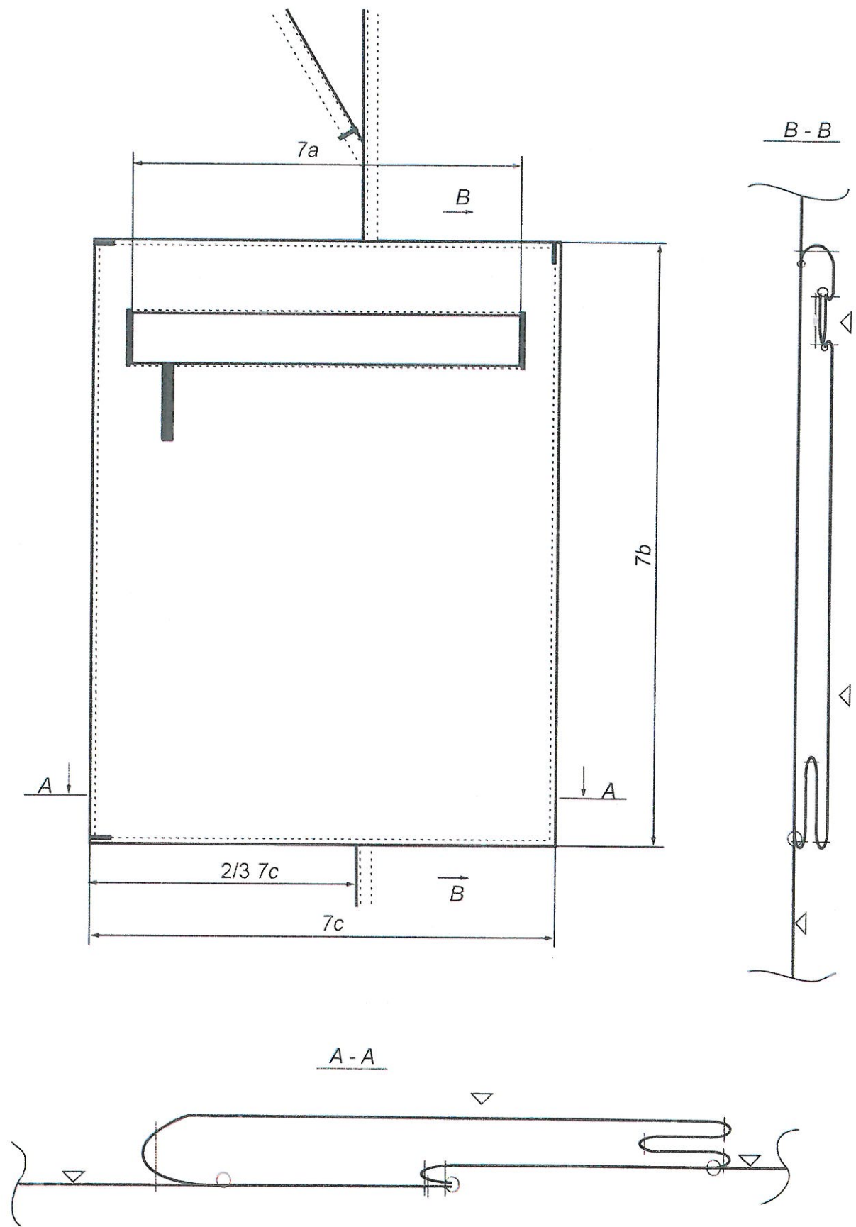
Rysunek 8 – Kieszęć udowa
